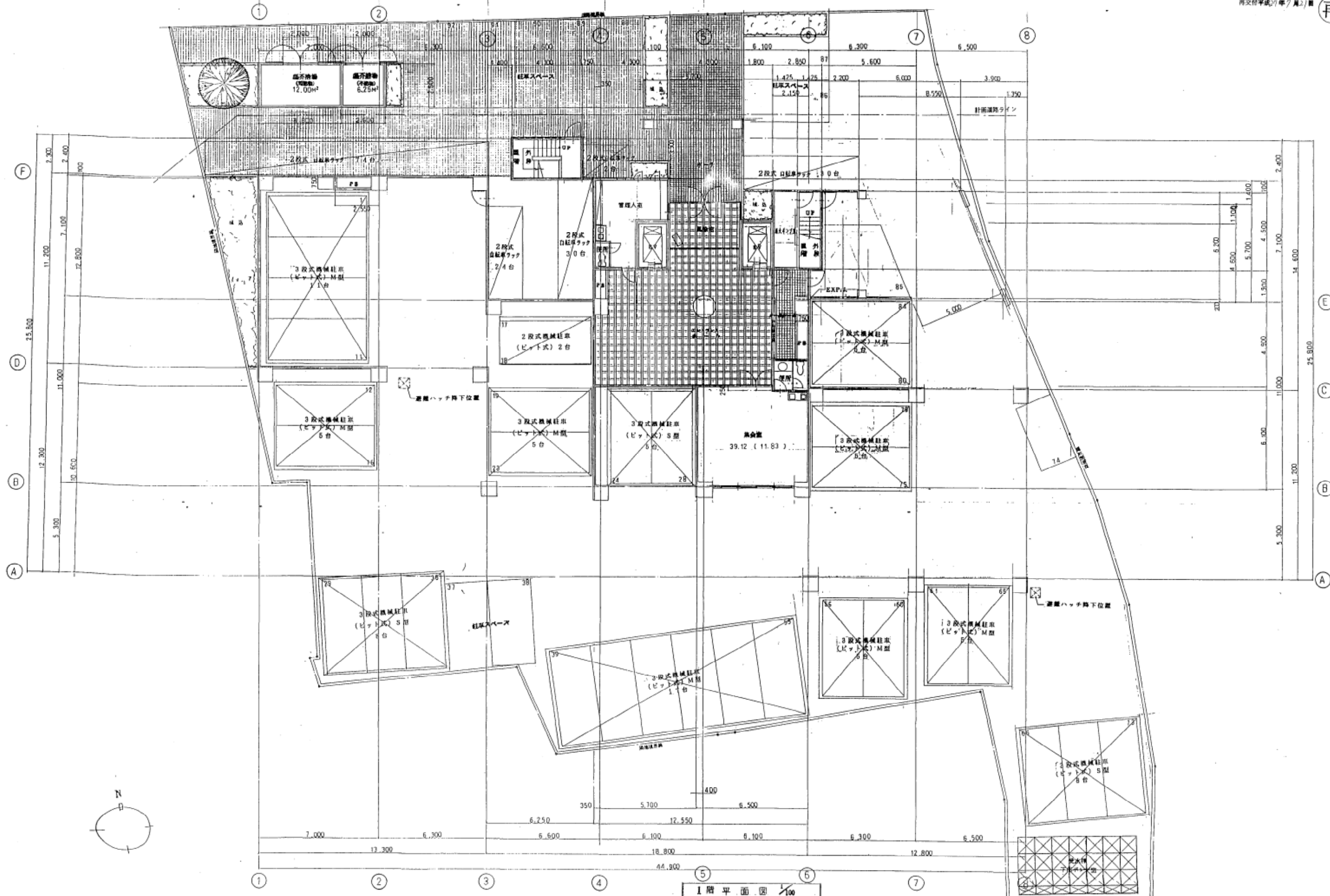
1F平面図
